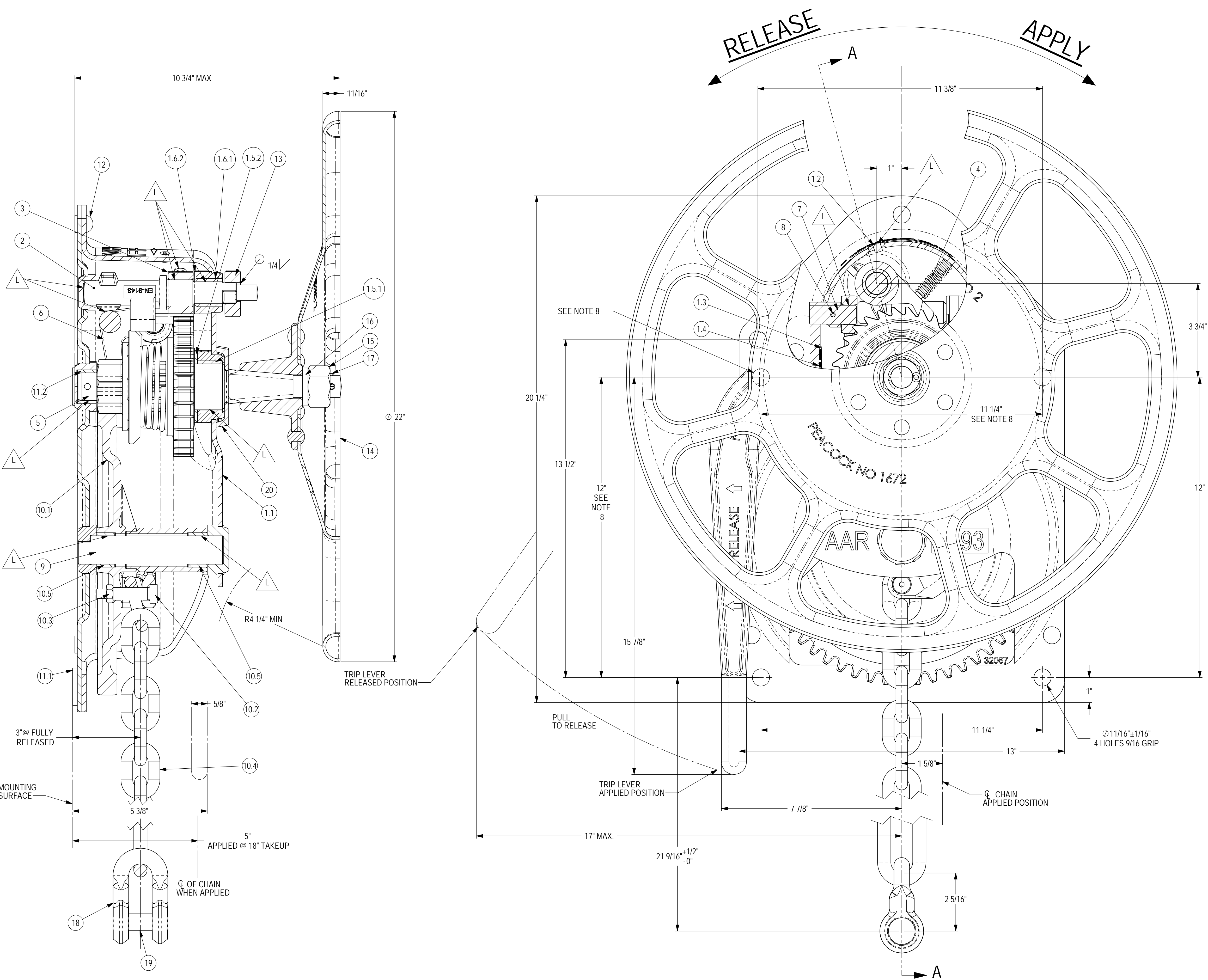
SECTION A-A
